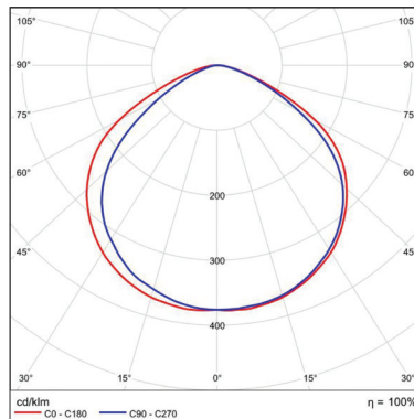
Fotometrijska krivulja 1SP SPF10W *
