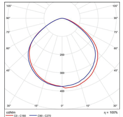
Fotometrijska krivulja 1SP SPF20W *
