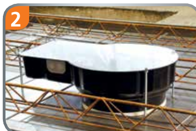
2 XXL Großdose auf den gewünschten Abstand schieben.
