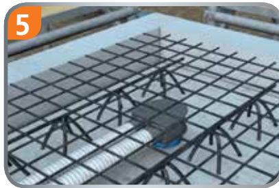
Rohre anschließen, obere Bewehrung einbringen und betonieren.
