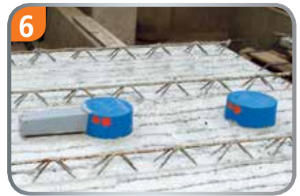
Betonfertigteil wird gegossen.
