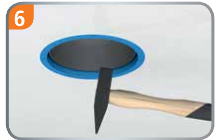
Lüftungshülse von unten mit Hammer einschlagen.
