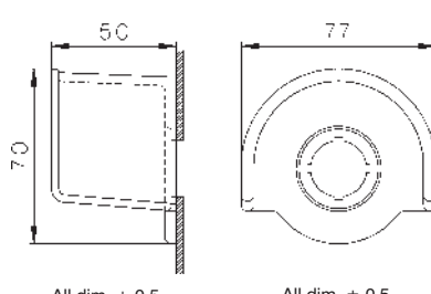
B3-SK ..
