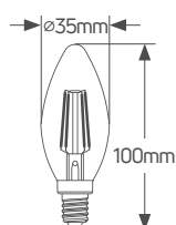
Vintage Candle 4W
