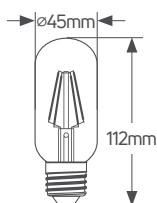
T45 Vintage 6W
