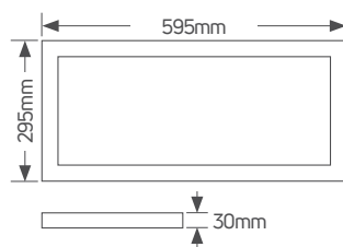
Panel Avra 60x30 UGR<19
