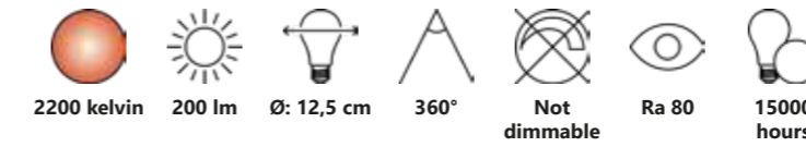
Amber 1428070 Glass
